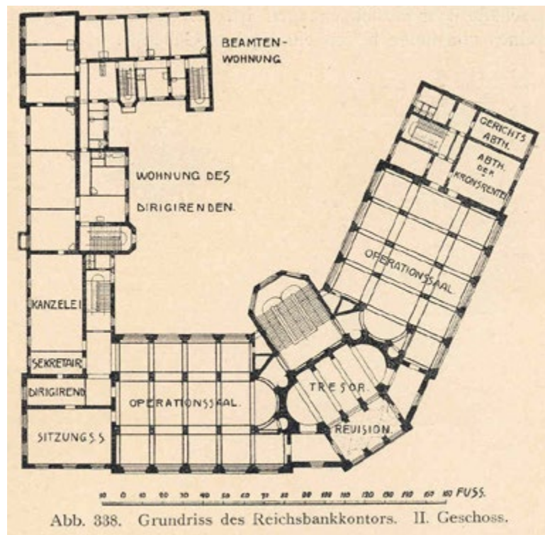
Bankas ēkas 2. stāva plāns, publicēts izdevumā "Riga und seine Bauten", 1905.
